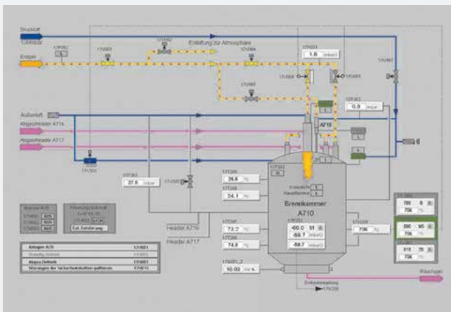
Prozessleittechnik: Bedienbilder für Brennersystem und Rauchgasreinigung
